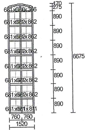
Poz. nr 9 Gabaryt 1520 x 6675 Ilość = 2
