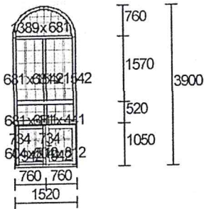
Poz. nr 10 WIEŻA Gabaryt 1520 x 3900 Ilość = 1
