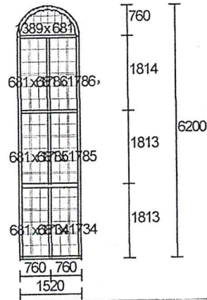
Poz. nr 11 WIEŻA Gabaryt 1520 x 6200 Ilość = 1
